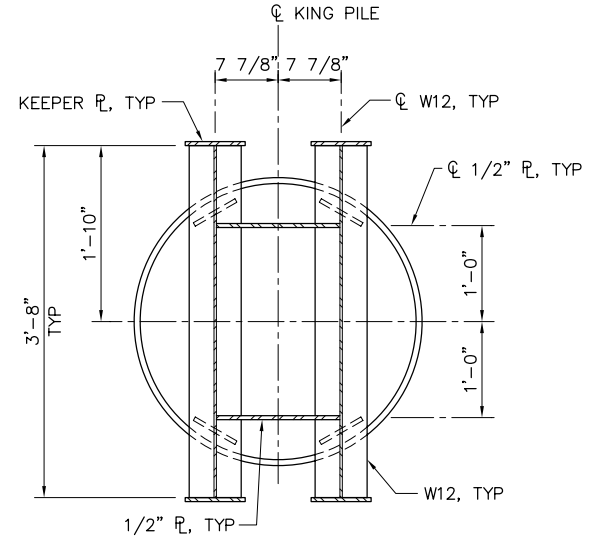
C SCALE: 1" = 1'-0"
