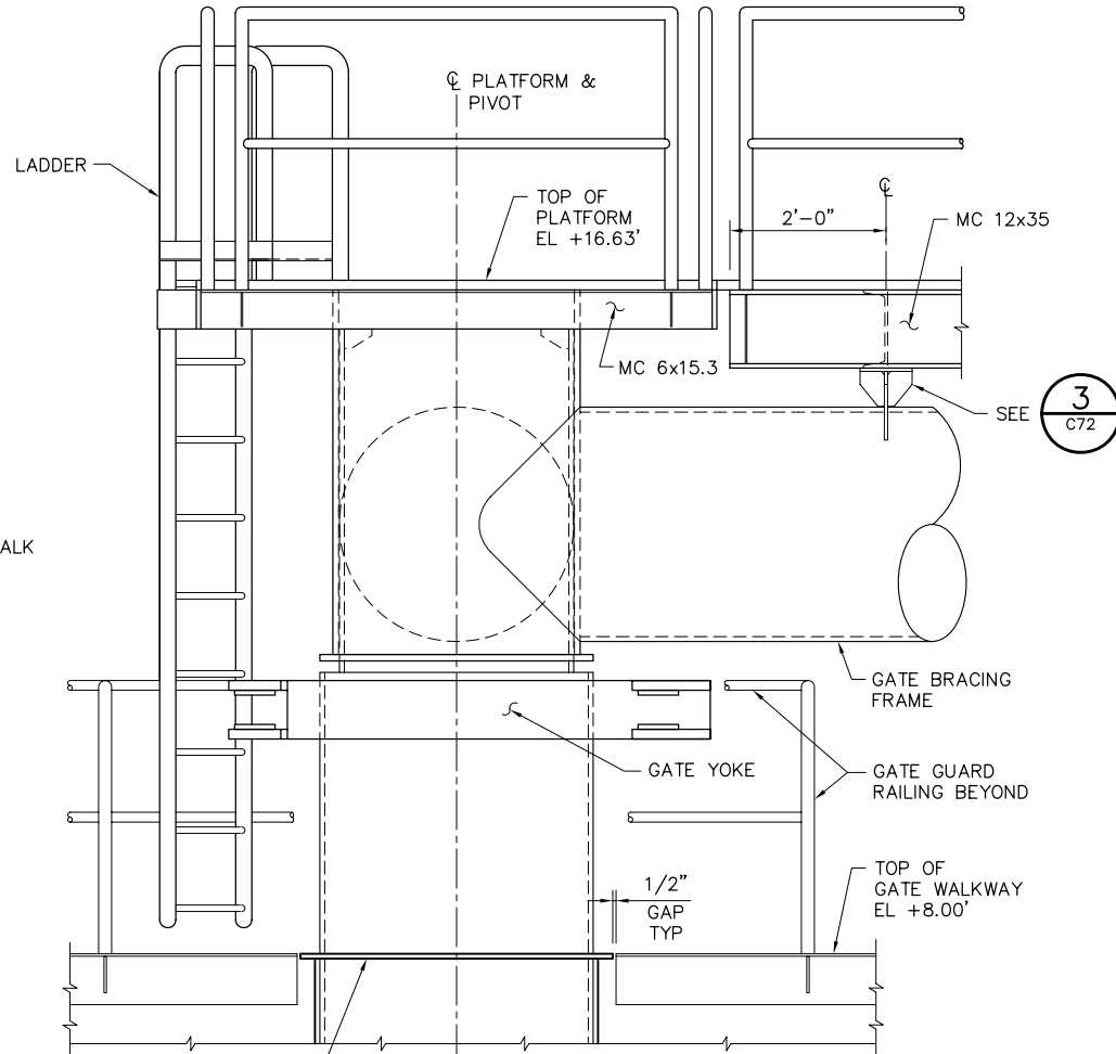
ELEVATION
