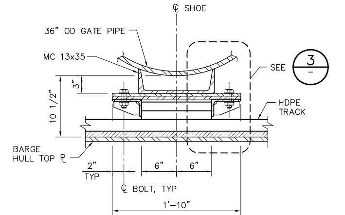
A SECTION SCALE: 1 1/2" = 1'-0"
