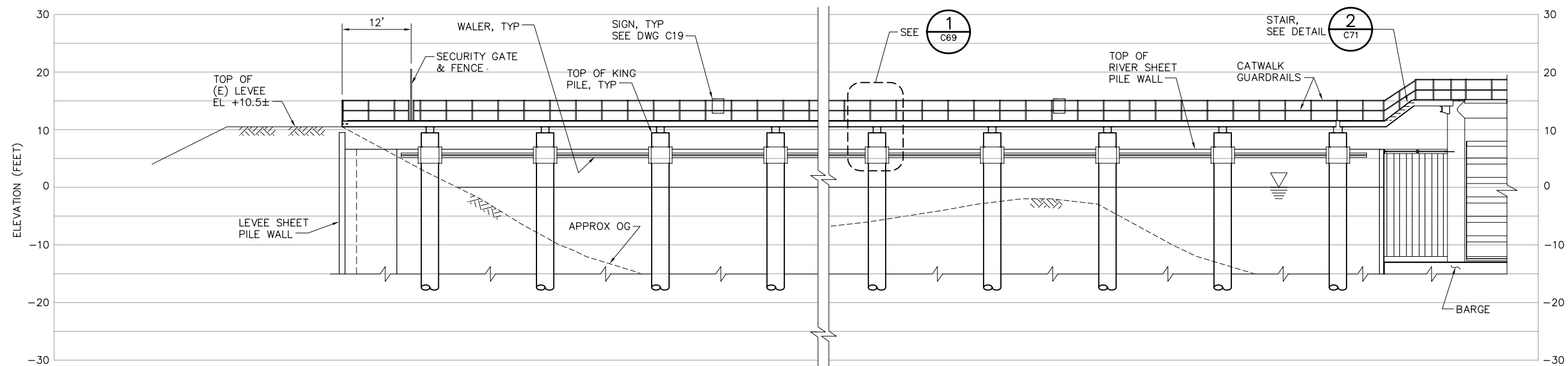
ELEVATION SCALE: 1"= 10'
