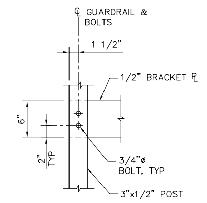
4 SCALE: 1 1/2" = 1'-0"
