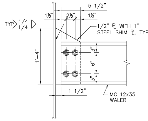
2 DETAIL SCALE: 1 1/2" = 1'-0"
