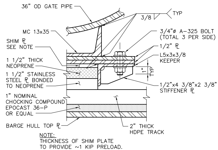
3 - DETAIL SCALE: 3" = 1'-0"
