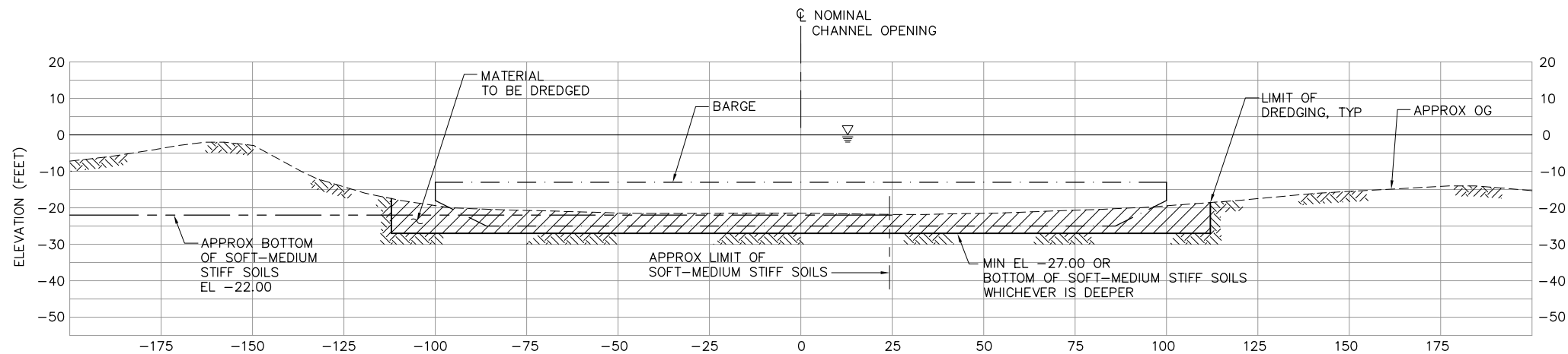
A SECTION SCALE: 1"=20'
