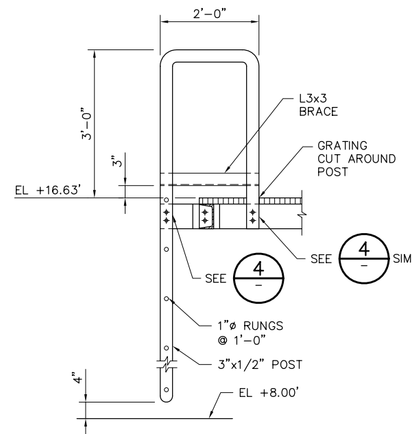
D SCALE: 3/4" = 1'-0"
