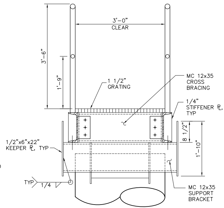
SECTION A SCALE: 1"=1'-0" C71
