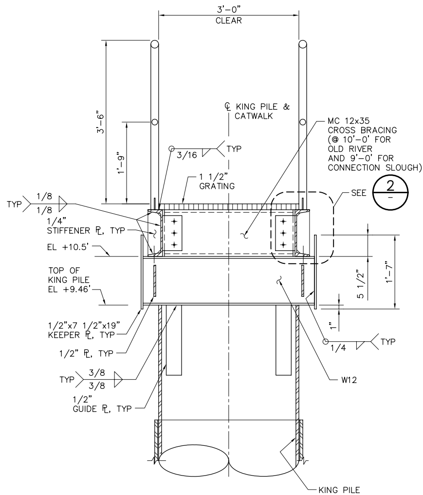
A SCALE: 1" = 1'-0"
