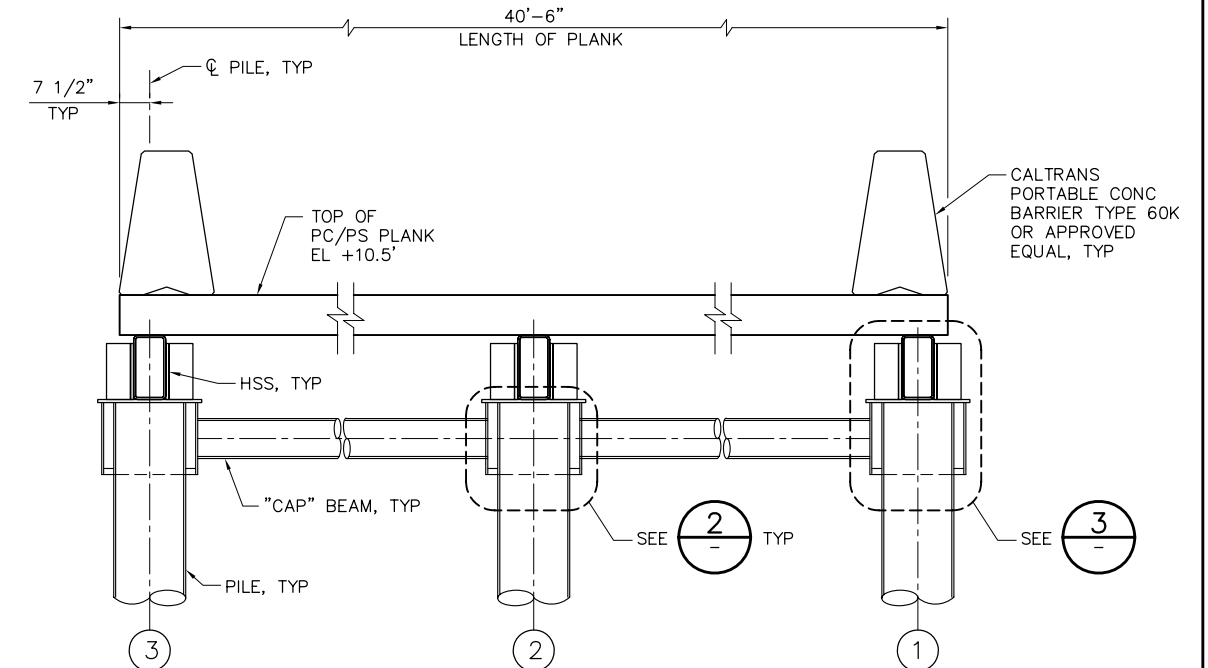
A SECTION SCALE: 1/2" = 1'-0"
