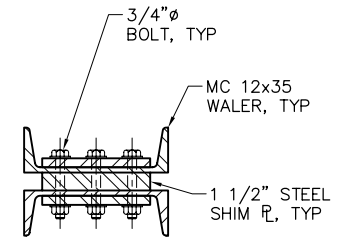
B SECTION SCALE: 1 1/2" = 1'-0"
