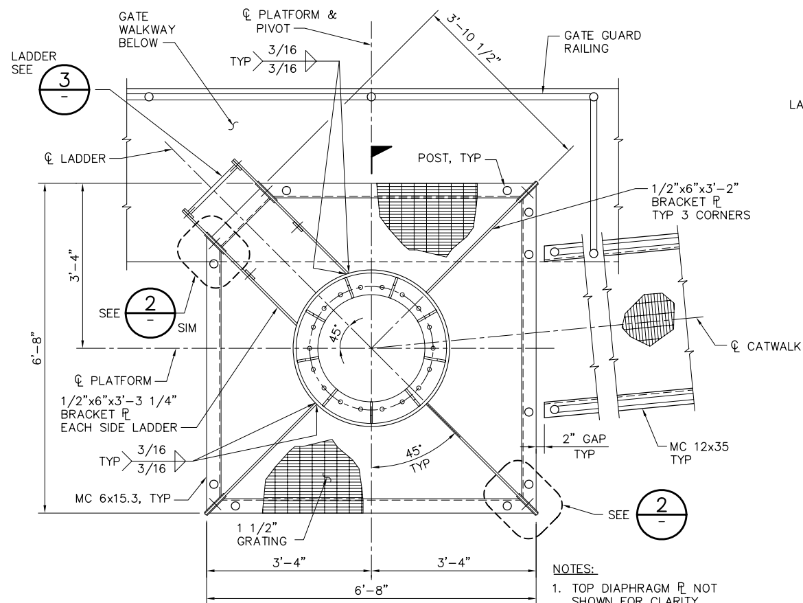
1 C14 SCALE: 3/4" = 1'-0"
