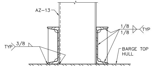
4 DETAIL SCALE: 1 1/2" = 1'-0"
