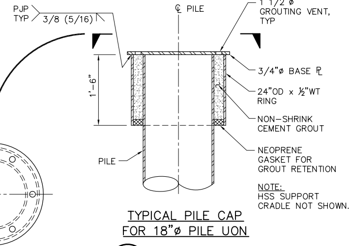
2 DETAIL SCALE: 1" = 1'-0"
