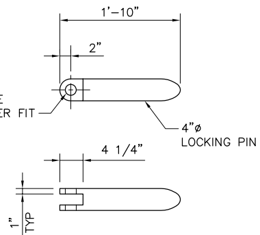
4 LOCKING PIN DETAIL SCALE: 1" = 1'-0"
