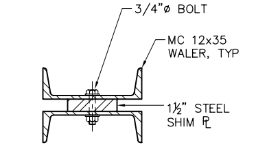
D SECTION SCALE: 1 1/2" = 1'-0"
