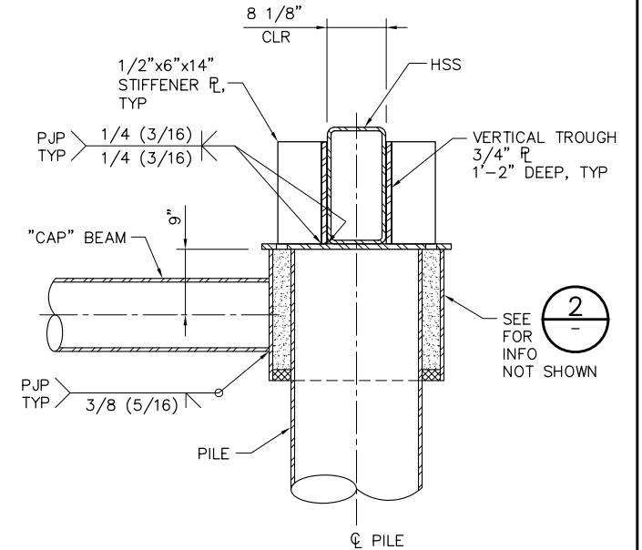
3 DETAIL SCALE: 1" = 1'-0"
