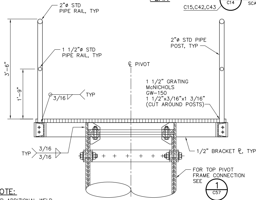
C SCALE: 1" = 1'-0"
