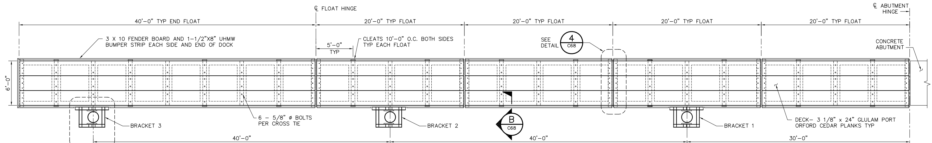
PLAN SCALE: 1/4" = 1'-0"
