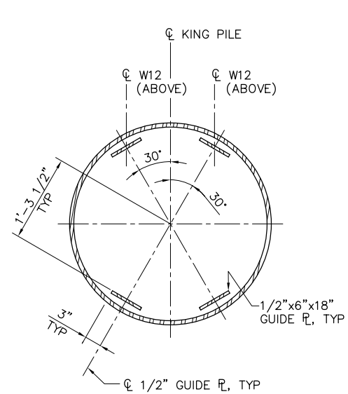
B SCALE: 1" = 1'-0"
