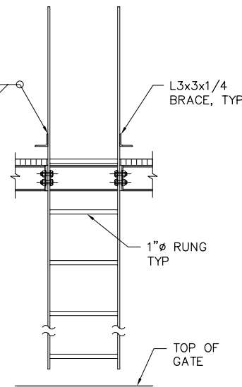
ELEVATION
