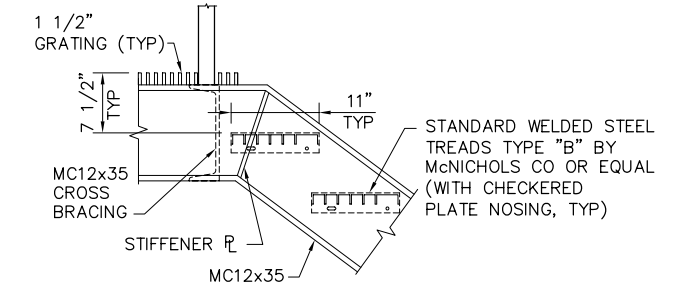
SECTION 4 SCALE: 1"=1'-0"
