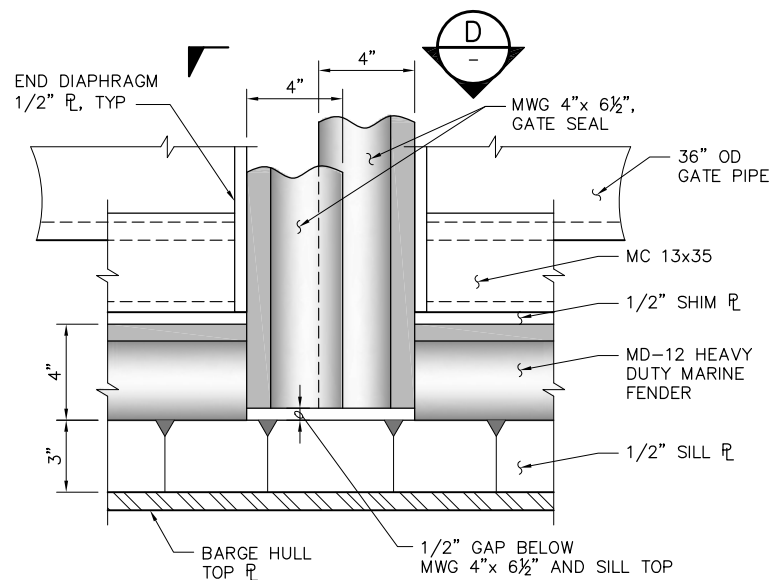
4 DETAIL C43 SCALE: 3" = 1'-0"
