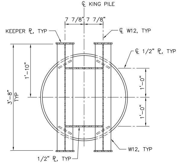
C SECTION SCALE: 1" = 1'-0"
