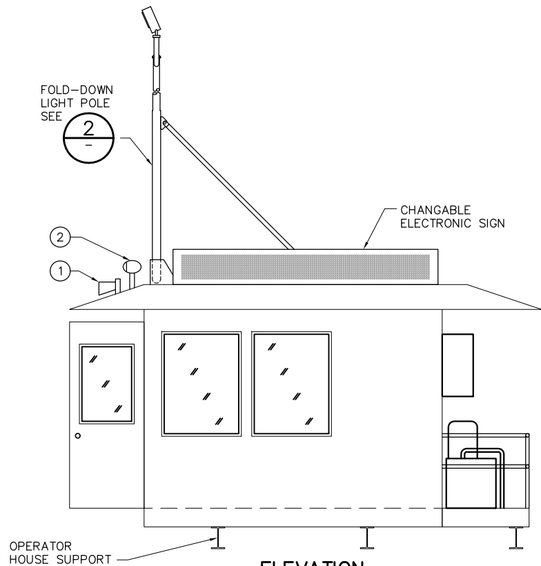
ELEVATION SCALE: 3/8" = 1'-0"
