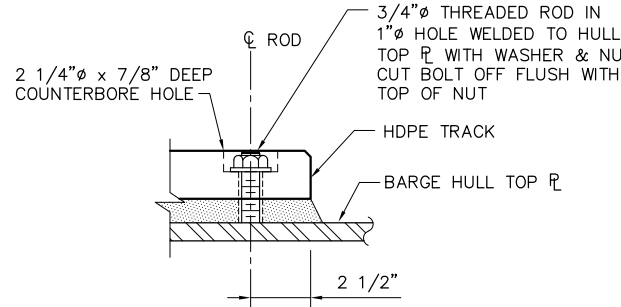
9 DETAIL SCALE: 3" = 1'-0"
