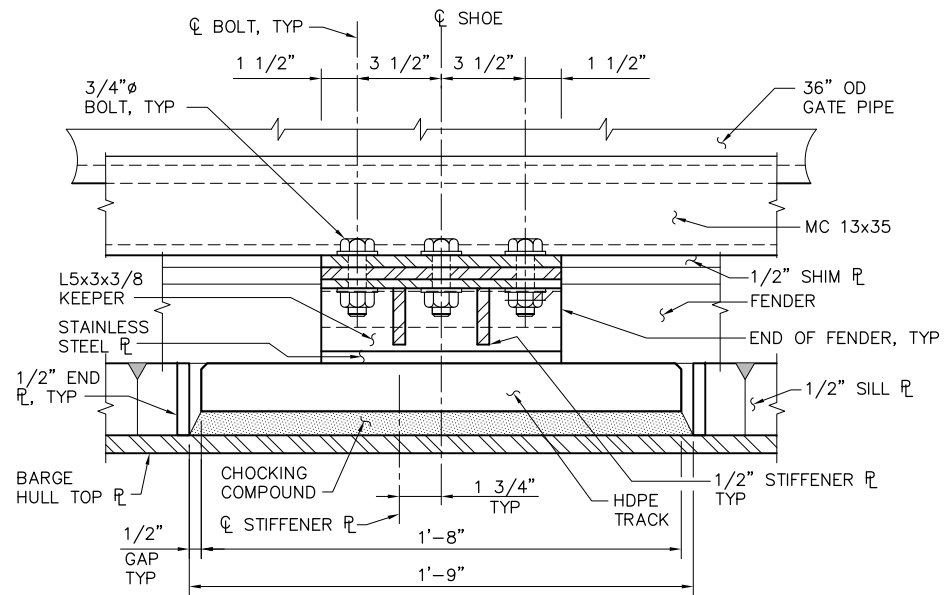
4 SECTION SCALE: 3" = 1'-0"
