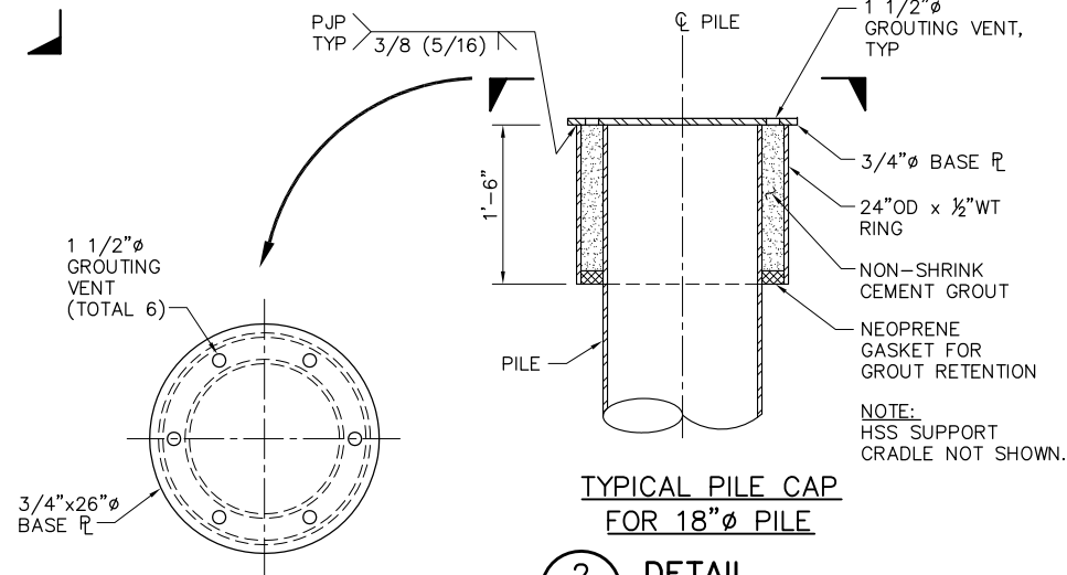
2 DETAIL SCALE: 1" = 1'-0"
