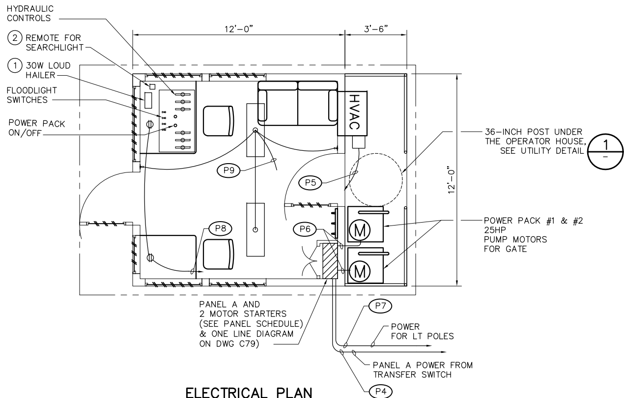
ELECTRICAL PLAN SCALE: 3/8" = 1'-0"
