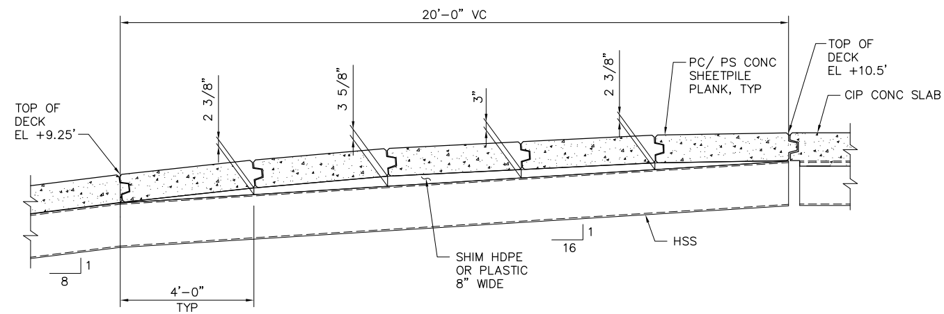
1 C7 DETAIL SCALE: 1/2" = 1'-0"
