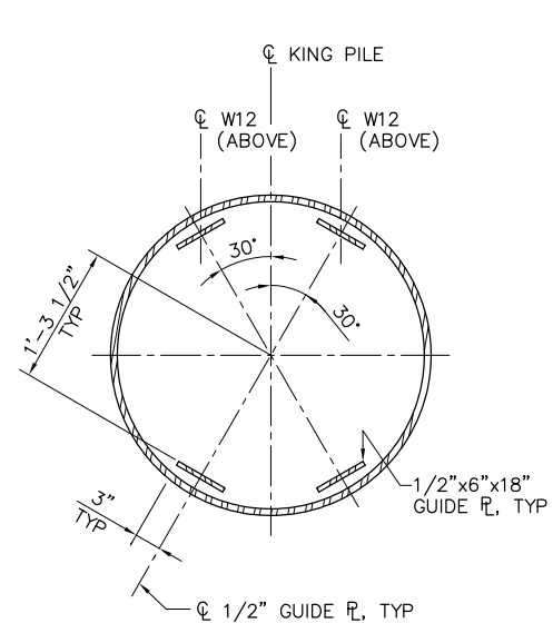
B SECTION SCALE: 1" = 1'-0"
