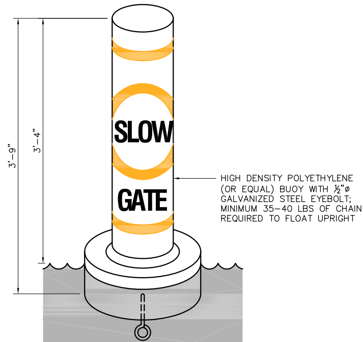
2 SLOW GATE SIGN C26 SCALE: 1/8" = 1'-0" C54
