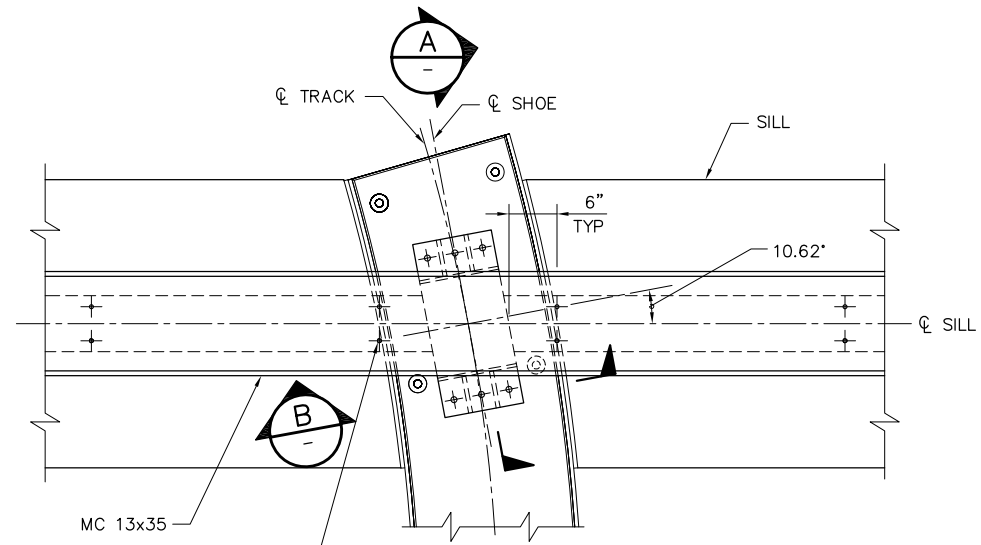
3 DETAIL SCALE: 1" = 1'-0"
