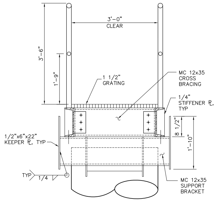
A SECTION C71 SCALE: 1" = 1'-0"
