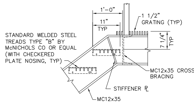
4 SCALE: 1"=1'-0"
