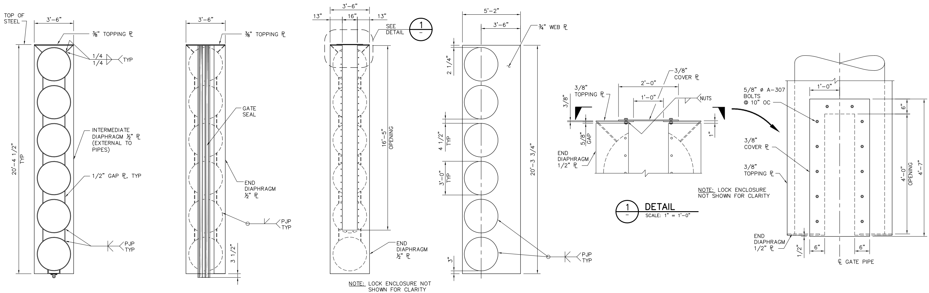
A SECTION C44 SCALE: 3/8"=1'-0"
