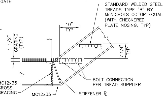
5 SCALE: 1"=1'-0"
