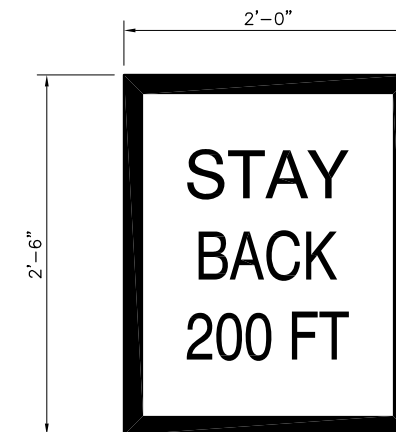
9 STAY BACK WARNING SIGN C26 SCALE: 1/8" = 1'-0" C54
