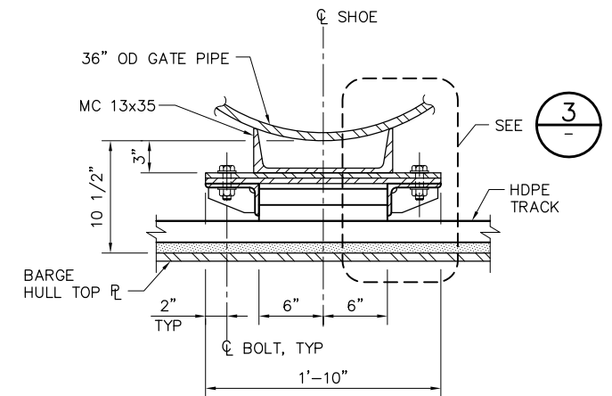
5 SECTION SCALE: 1 1/2" = 1'-0"
