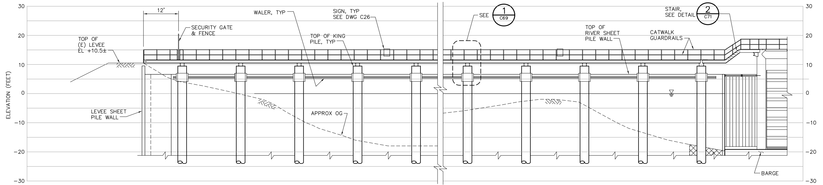
ELEVATION SCALE: 1"= 10'
