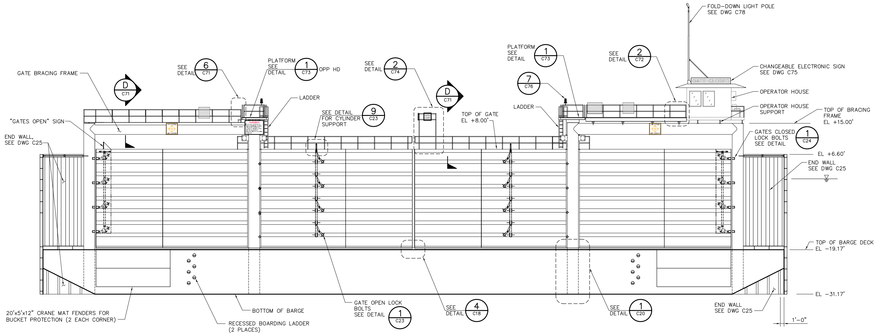
ELEVATION SCALE: 1/8"= 1'-0"
