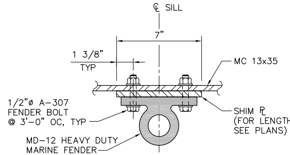
7 DETAIL SCALE: 3" = 1'-0"
