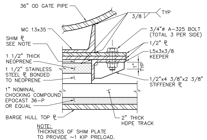
6 DETAIL SCALE: 3" = 1'-0"
