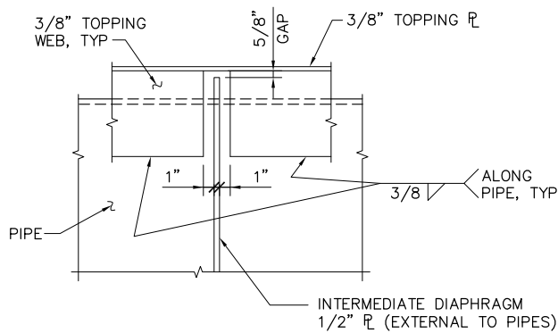
3 DETAIL C44 SCALE: 1 1/2" = 1'-0"
