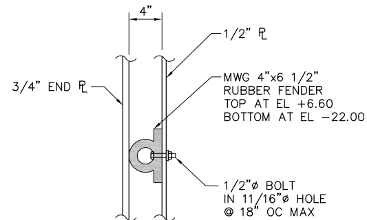
4 DETAIL SCALE: 1 1/2" = 1'-0"
