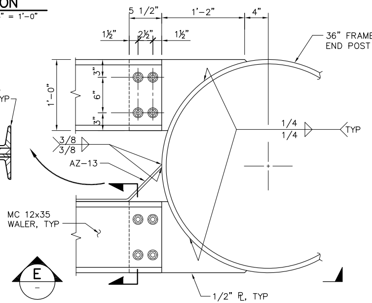
3 DETAIL SCALE: 1 1/2" = 1'-0"
