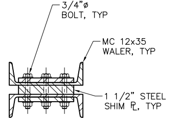
B SECTION SCALE: 1 1/2" = 1'-0"
