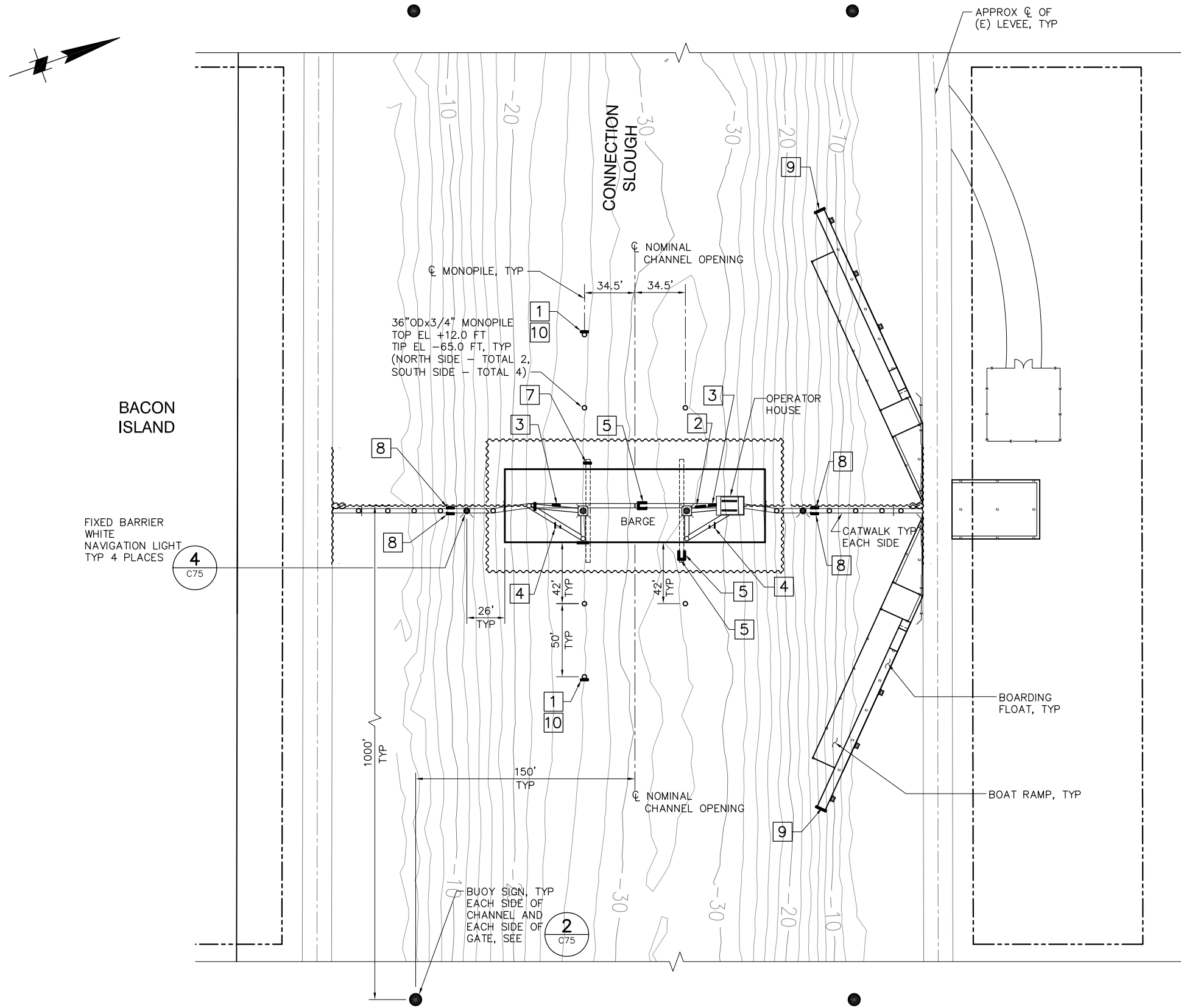
PLAN SCALE: 1"= 40'
