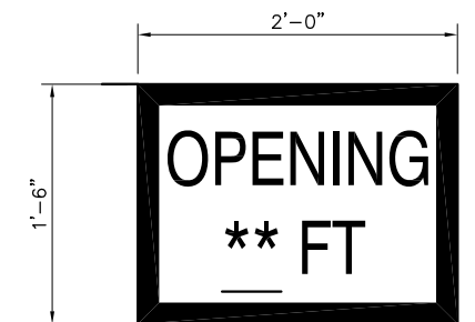
8 ELECTRONIC MESSAGE SIGN C26 SCALE: NONE C54
