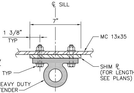
7 DETAIL SCALE: 3" = 1'-0"
