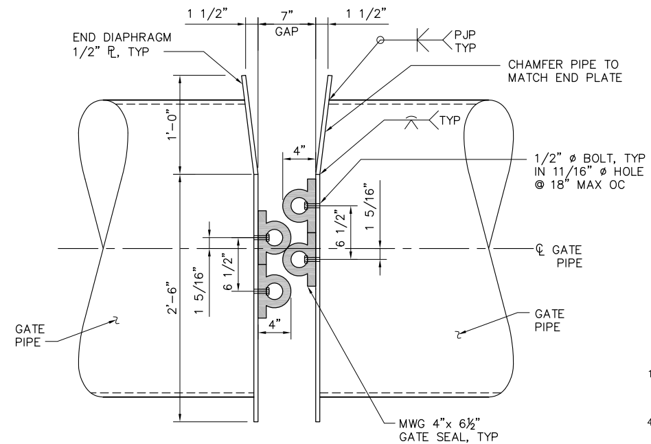
D SECTION SCALE: 1 1/2" = 1'-0"
