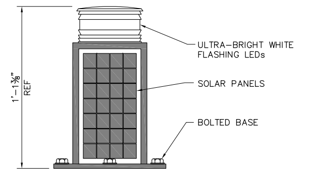
4 NAVIGATION LIGHT C26 SCALE: NONE C54
