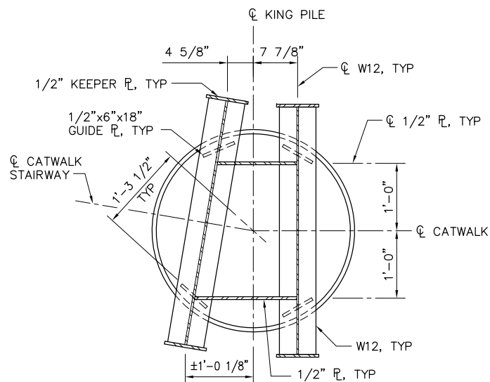
3 DETAIL SCALE: 1" = 1'-0"
