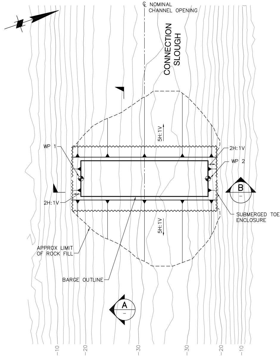
PLAN SCALE: 1"= 40'
