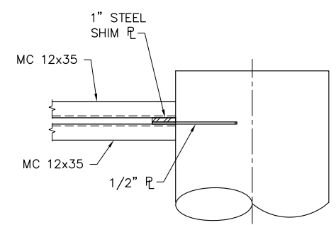
E SECTION - SCALE: 3/4"=1'-0"
