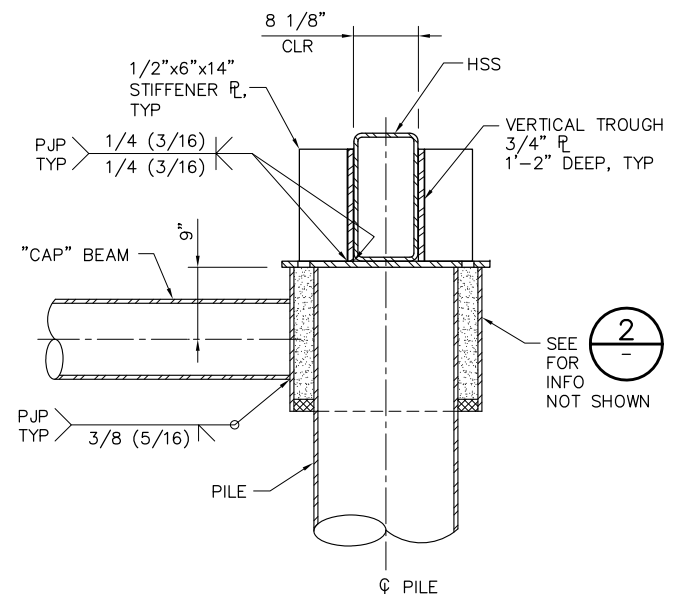
3 DETAIL SCALE: 1" = 1'-0"
