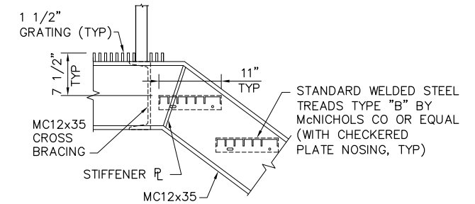
4 DETAIL SCALE: 1" = 1'-0"
