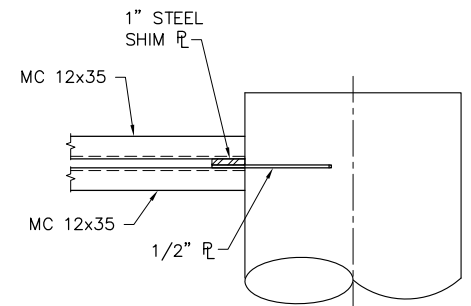
E SECTION SCALE: 3/4" = 1'-0"
