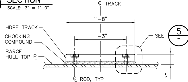
8 SECTION SCALE: 1 1/2" = 1'-0"
